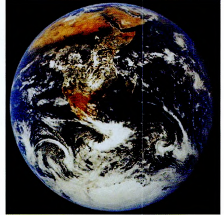
Планета Зямля
