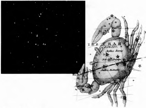
Сузор'е Рака
