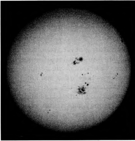
Сонца з плямамі
