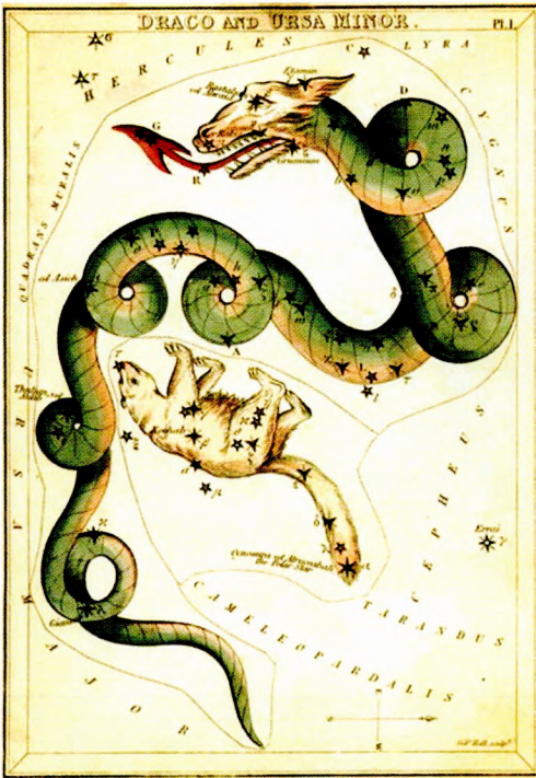
Вьява сузор'яў Дракона, Малой Мядзведзіцы ў атласе 1825 года Дж. Аспін
