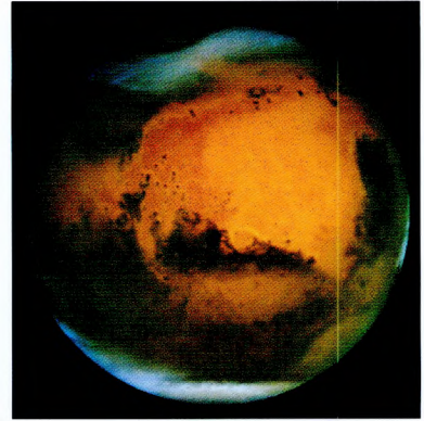
Планета Марс
