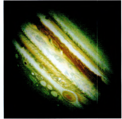
Планета Юпітэр
