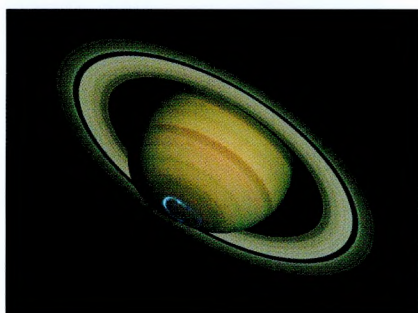
Сатурн
