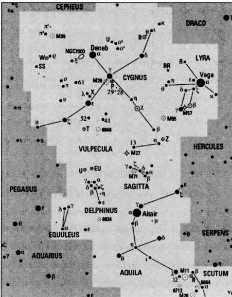
Карта з сузор'ямі Лебедзя, Ліры, Арла, Лісічки, Стрالی, Дельфіна
