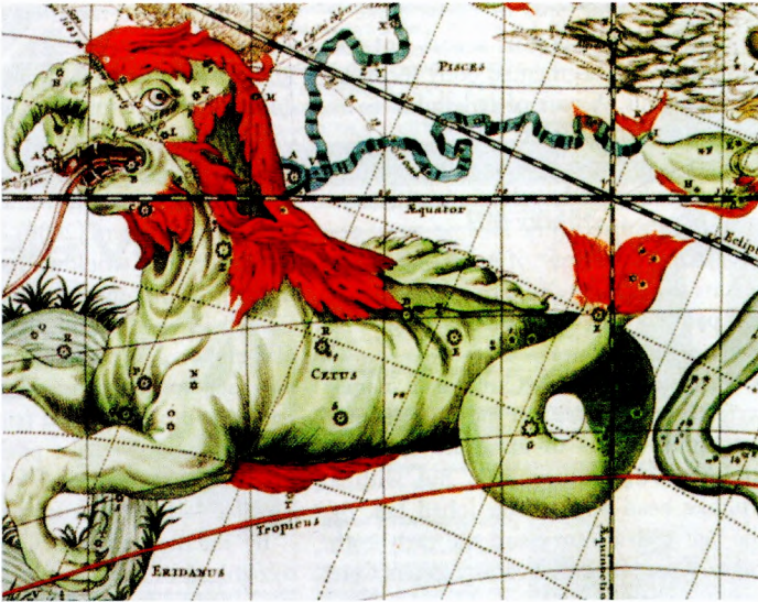
Вьява сузор'я Кита. Малюнак з кнігі 1729 г.
