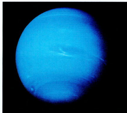
Планета Нептун
