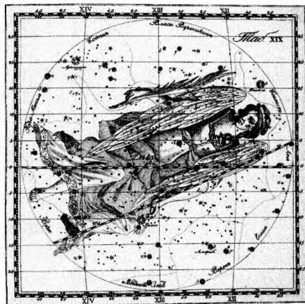
Выява сузор'я Дзевы ў атласе Карнелія Рэйсіса. 1829
