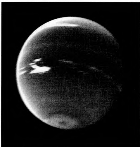
Нептун
