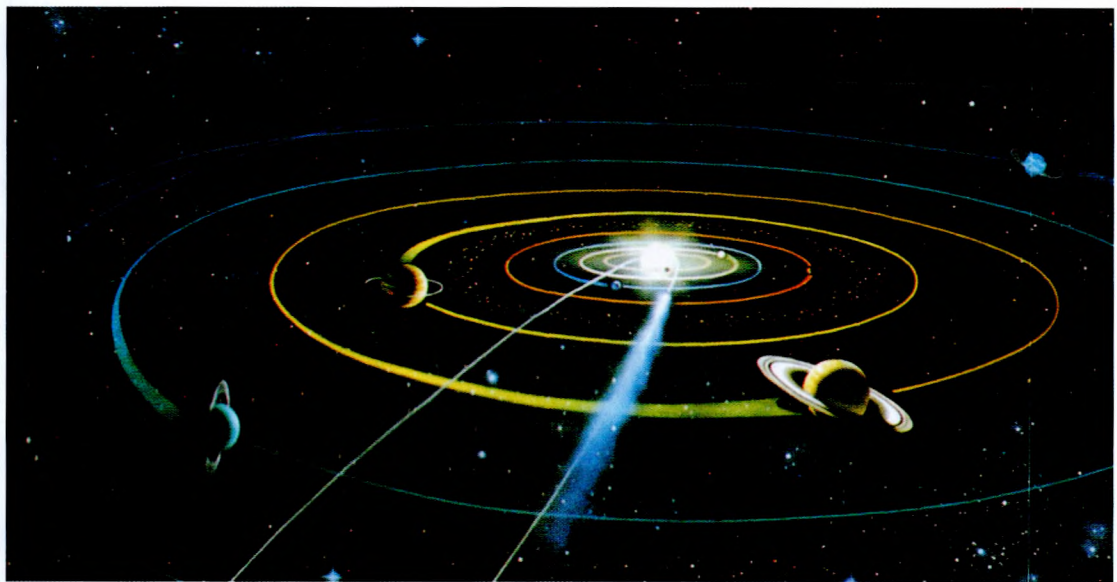
Сонечная сістэма
