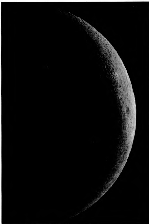
Растучы Месяц
