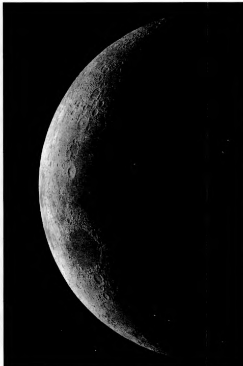
Убываючы Месяц
