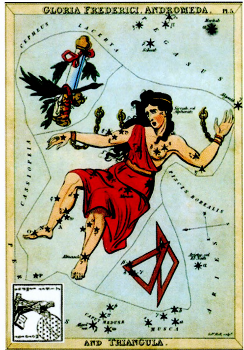
Вьява сузор'яў Андромеды і Трыкутніка ў атласе 1825 года Дж.Аспін
