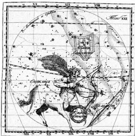
Сузор'е Стральца ў атласе Карнеля Рэйсіса. 1829
