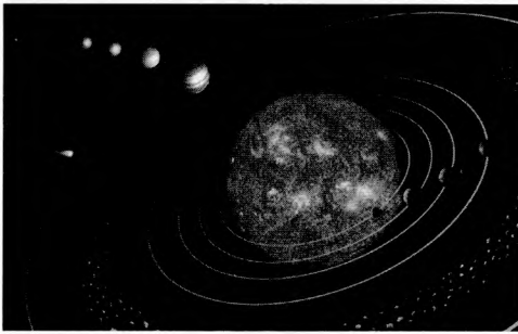
Сонечная сістэма
