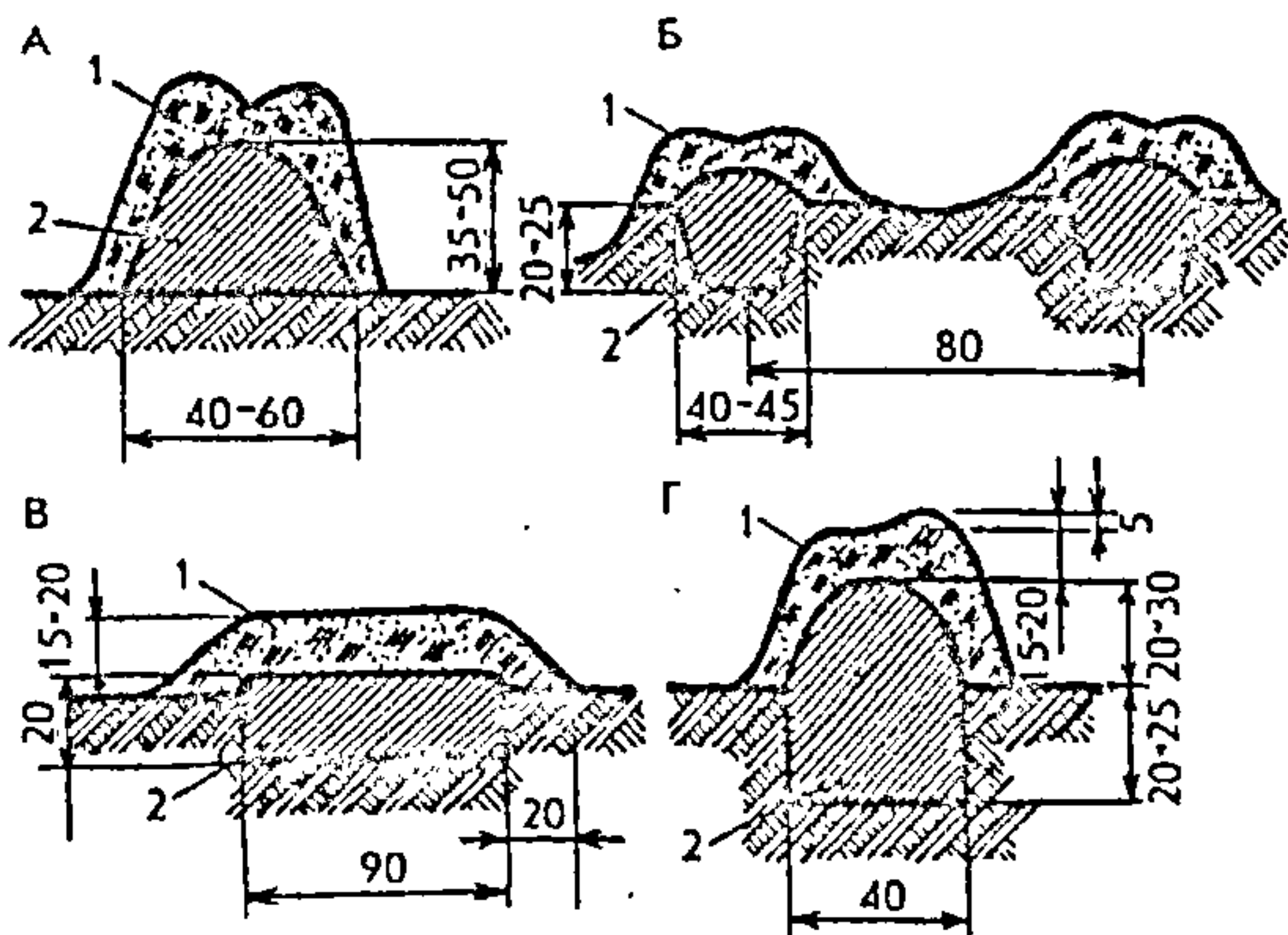
Мал. 12. Уцеплены грунт без пакрыцця на біялагічным наліве (памеры ў сантыметрах):
