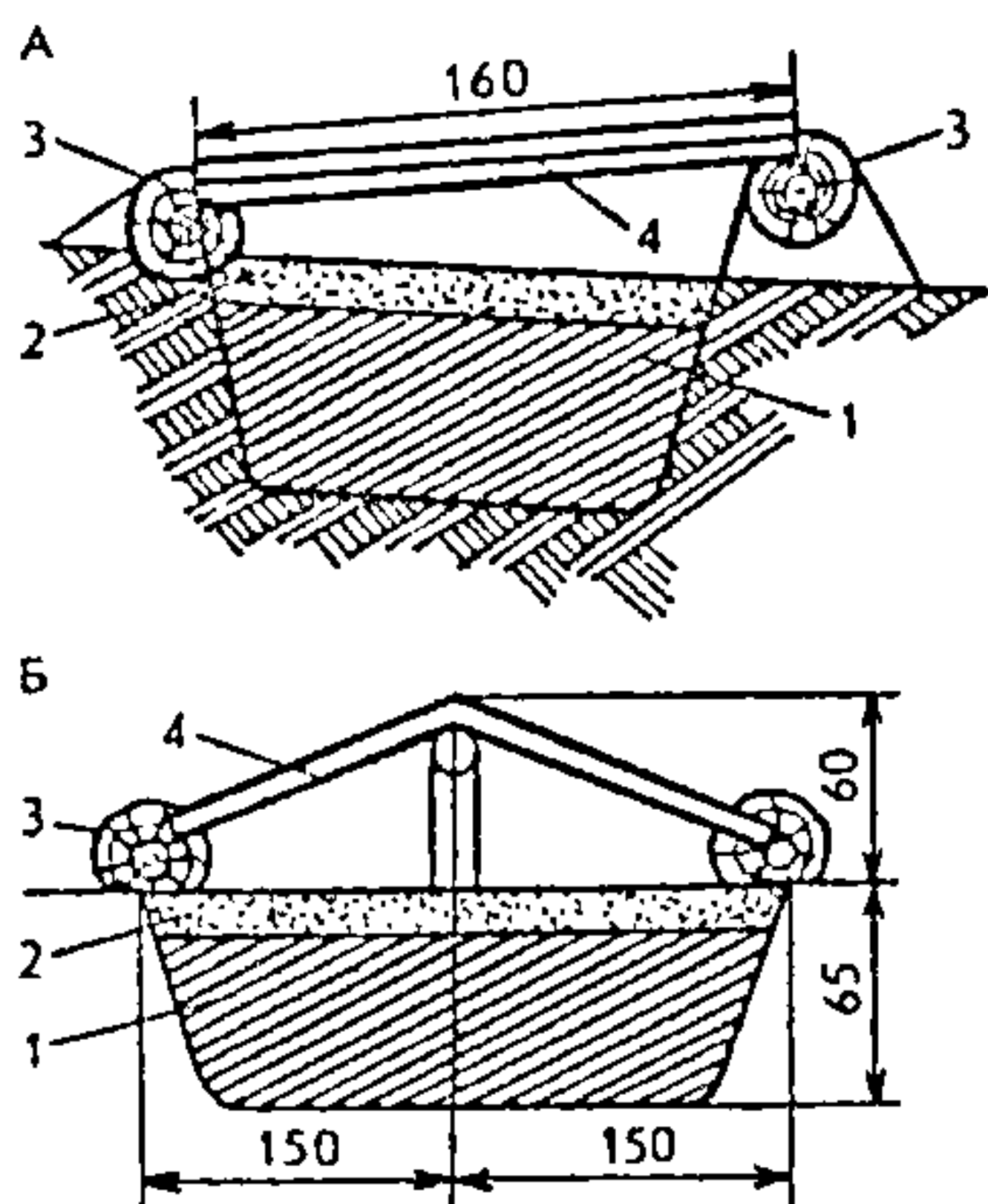
Мал. 10. Парнікі. А – аднаскатны, Б – двухскатны: 1 – біяпаліва; 2 – грунт; 3 – парубень; 4 – парніковая рама (памеры ў сантыметрах).
