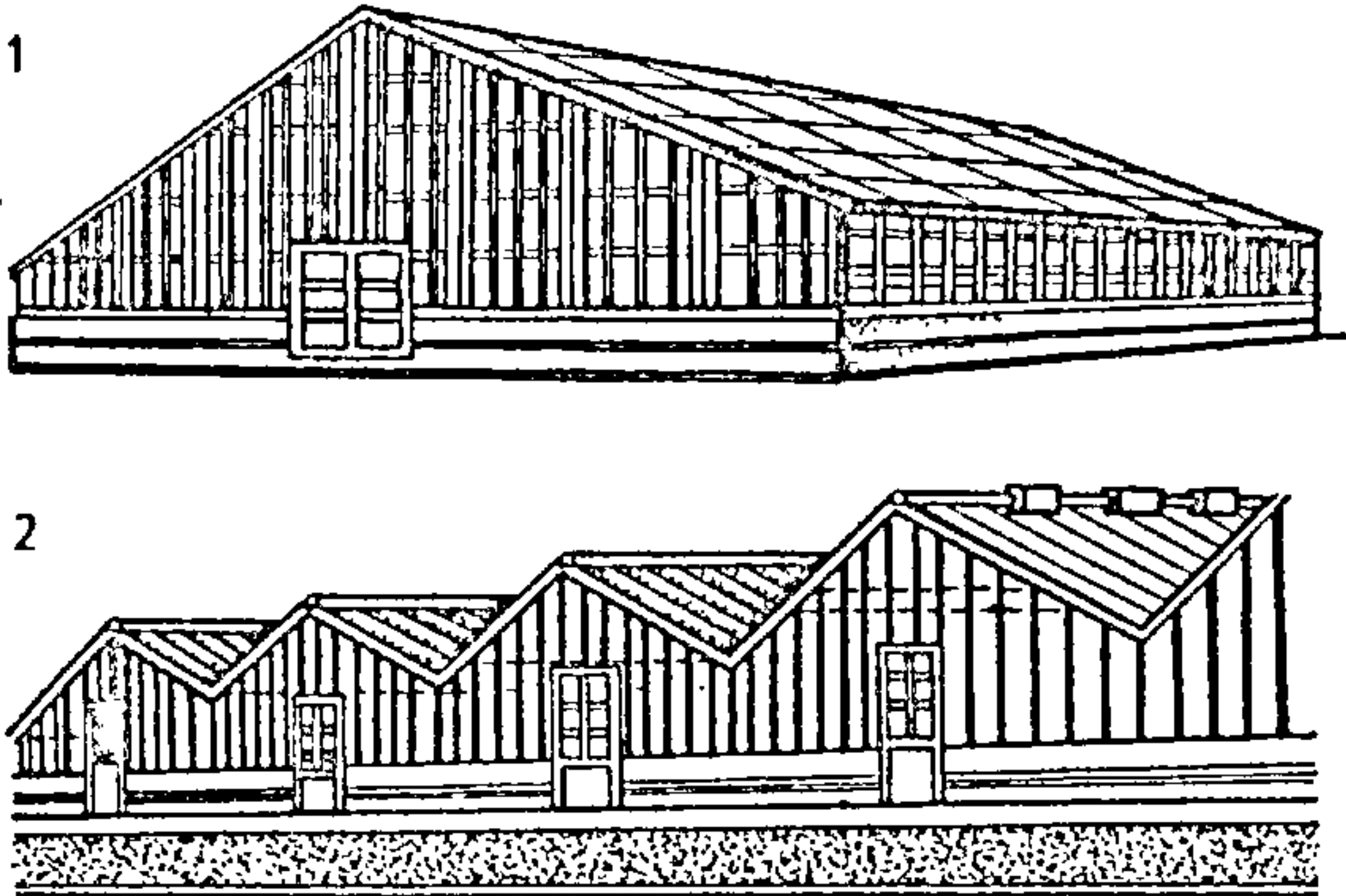
Мал. 9. Тыпы цяпліц: 1 – ангарная; 2 – блочная.
