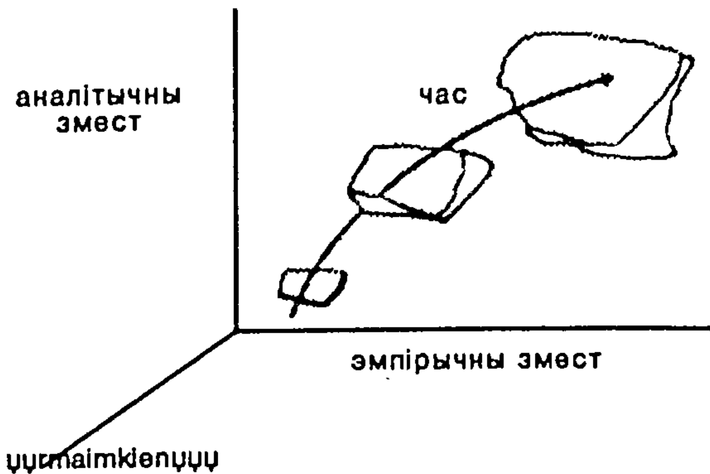
Трохмерная сістэма каардынат Холтана
