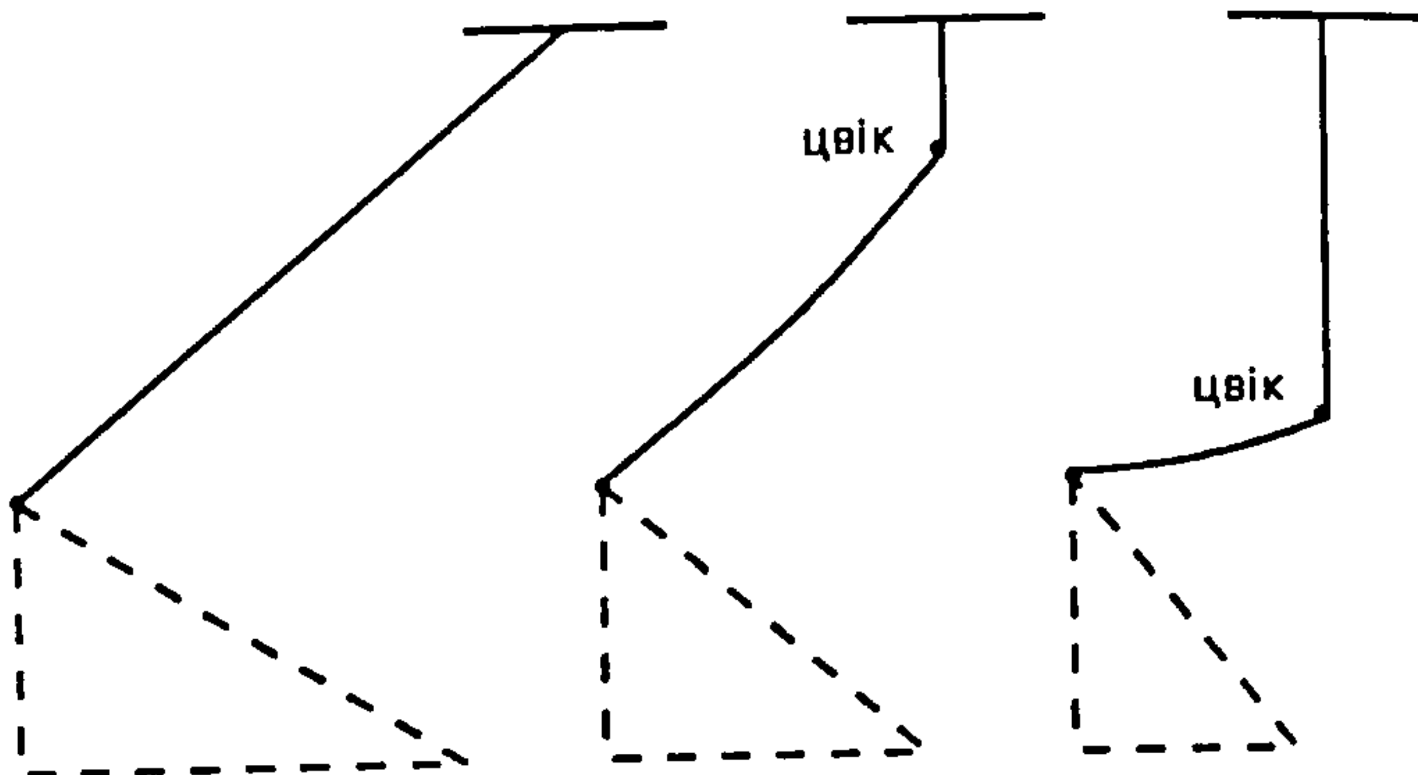
Эксперымент Галілея з маятнікам і цвіком
