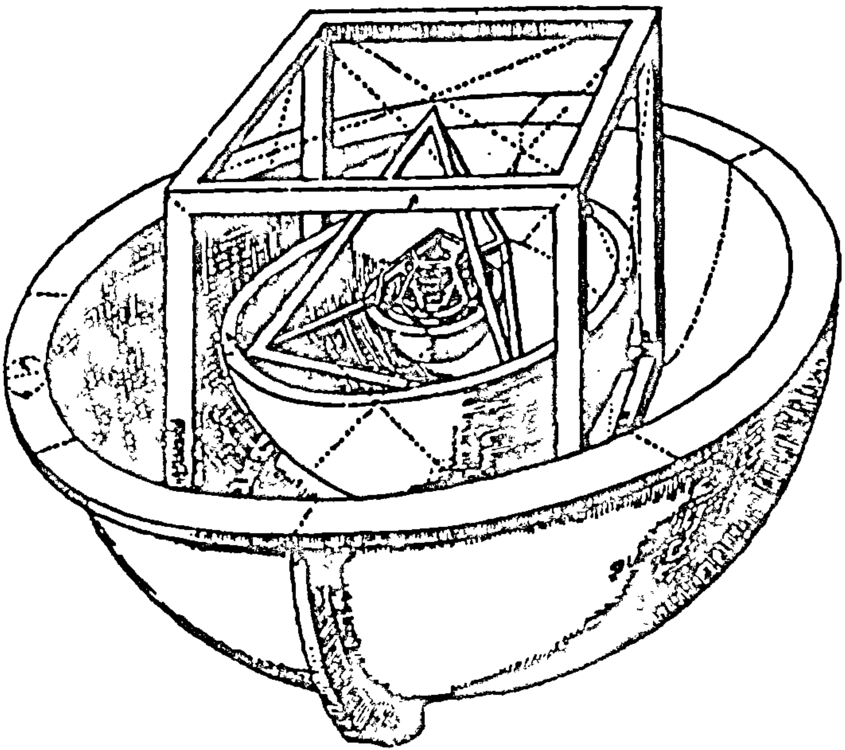
Кеплераўская сістэма правільных геаметрычных целаў
