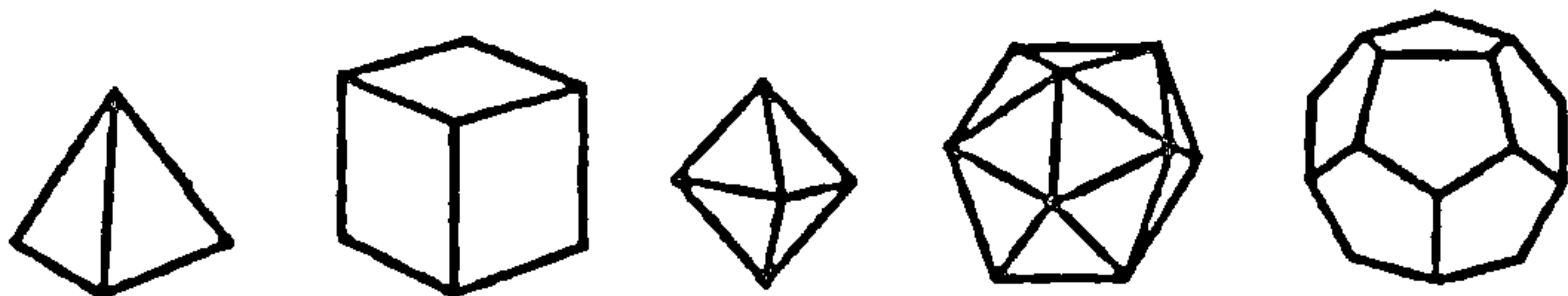
Дадэкаэдр (нябеснае рэчыва)
